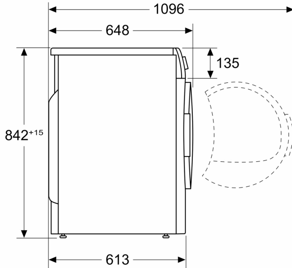
Matmenys, mm
