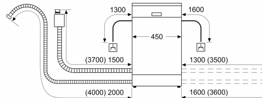
matmenys mm
