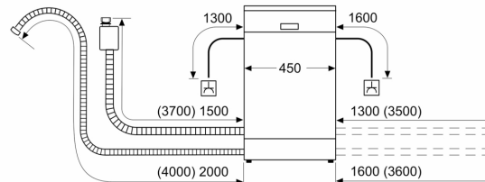
matmenys mm
