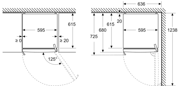
Matmenys, mm
