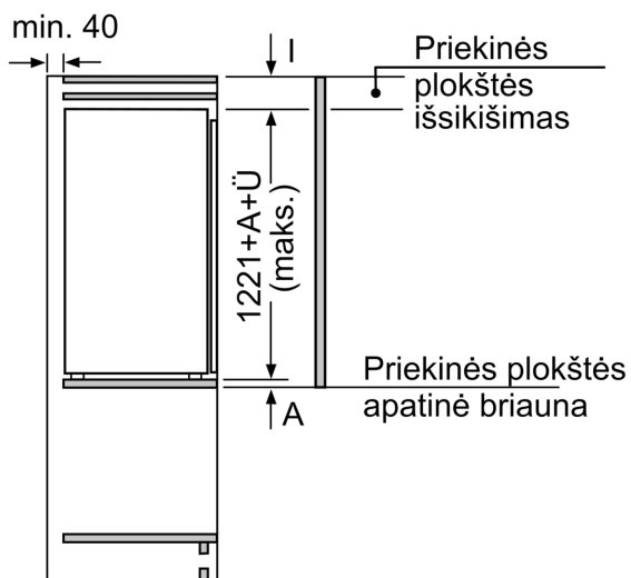
Matmenys, mm
