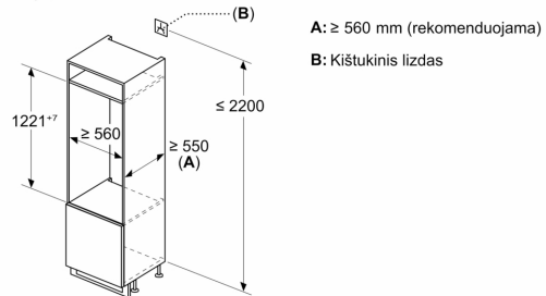
Matmenys, mm
