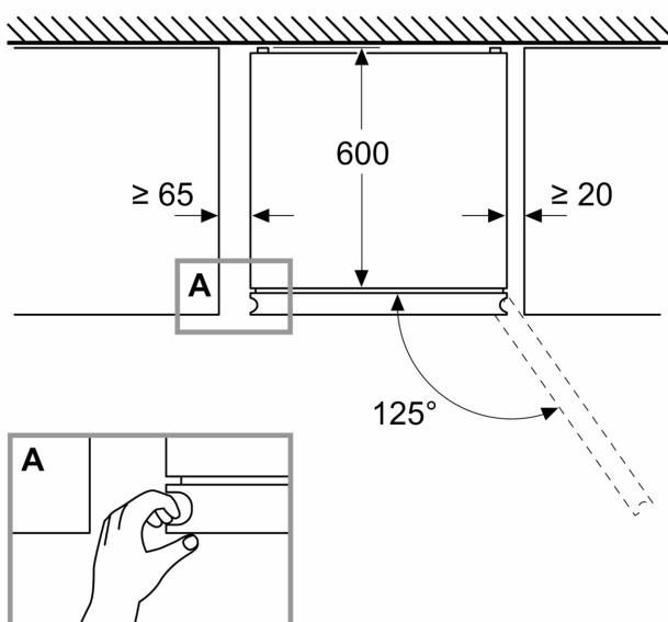
Matmenys, mm
