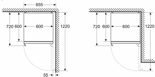
Matmenys, mm
