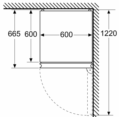
Matmenys, mm
