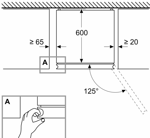
Matmenys, mm
