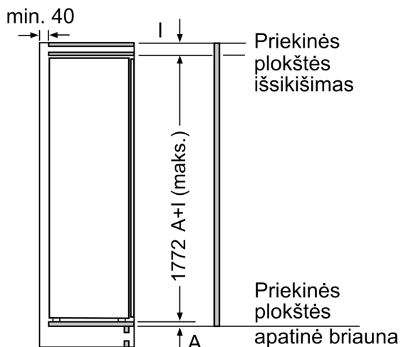
Matmenys, mm
