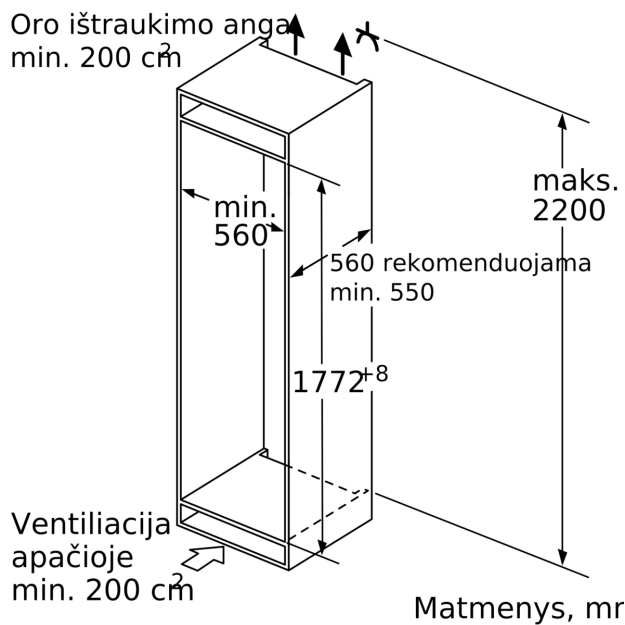
Matmenys, mm
