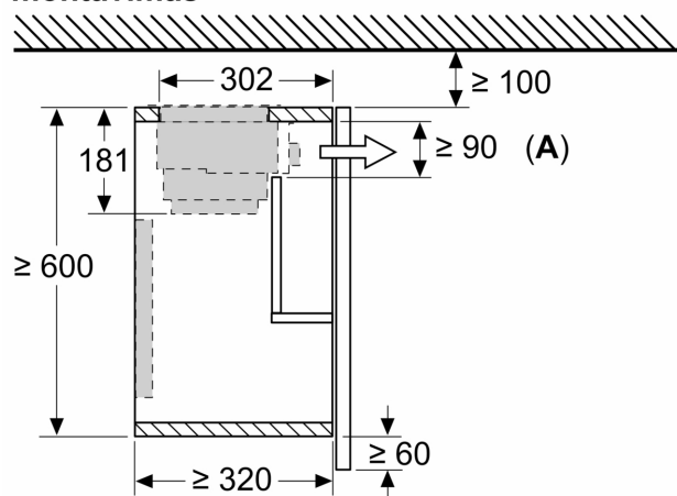
Matmenys, mm Ištraukiamojo gartraukio su recirkuliacijos rinkiniu ir nuleidžiamuoju rėmu montavimas
