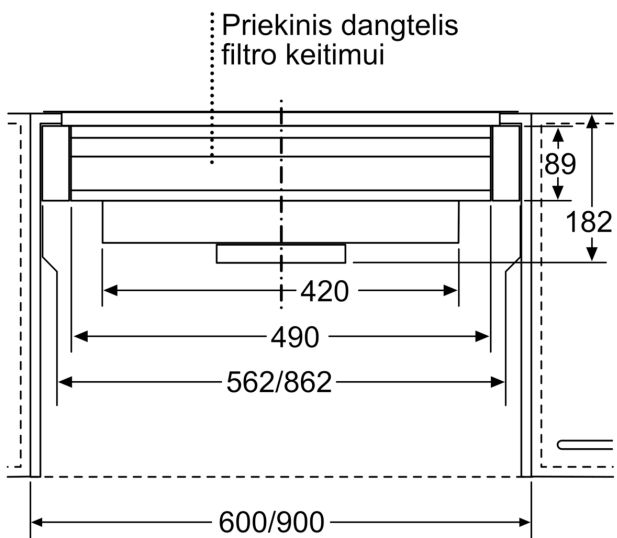
Matmenys, mm
