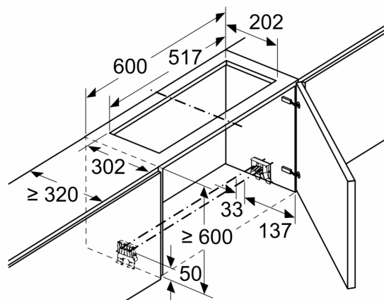
Matmenys, mm Ištraukiamojo gartraukio su recirkuliacijos rinkiniu montavimas
