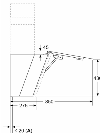
Matmenys, mm
