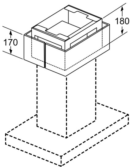
Matmenys, mm
