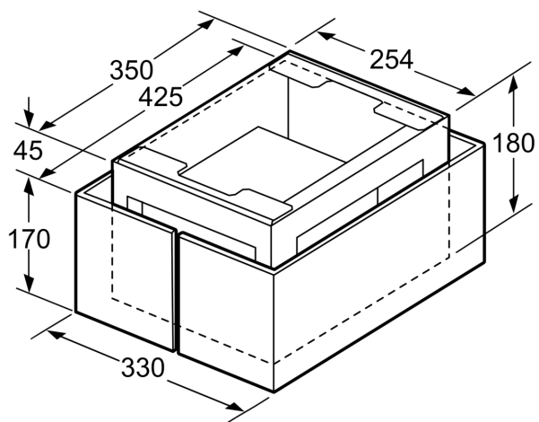
Matmenys, mm
