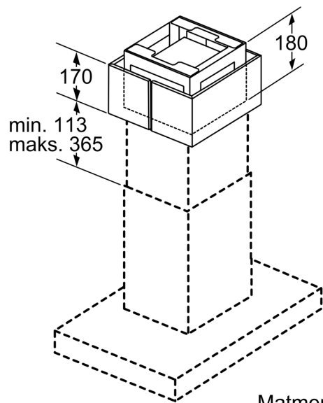
Matmenys, mm
