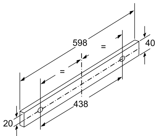
Matmenys, mm
