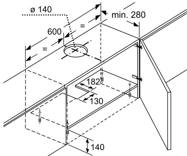
Matmenys, mm
