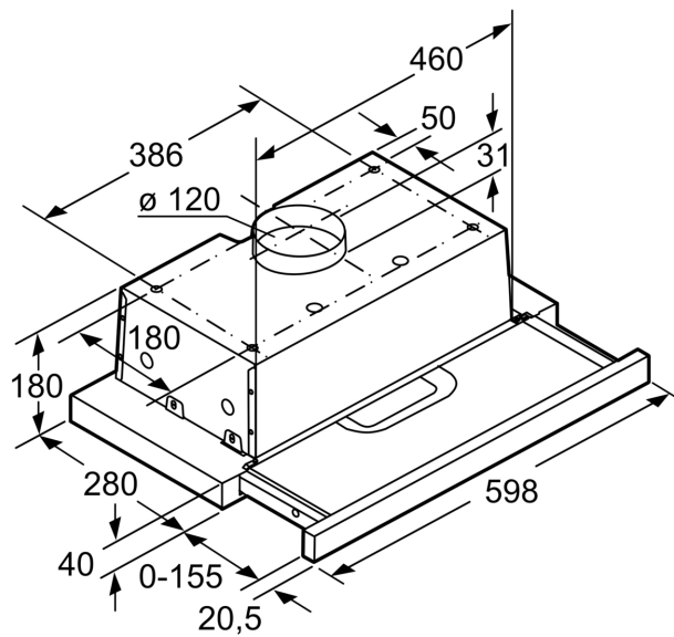
Matmenys, mm
