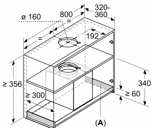
Matmenys, mm Montavimo pavyzdys
