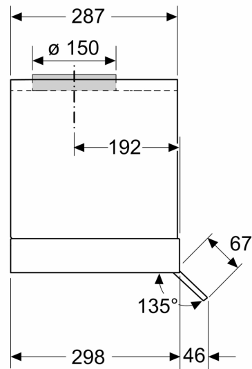
Matmenys, mm Vaizdas iš šono
