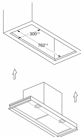
Matmenys, mm Montavimo pavyzdys su baldo išpjova
