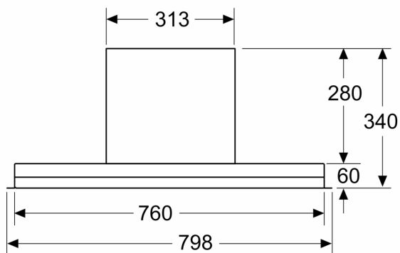
Matmenys, mm Vaizdas iš priekio
