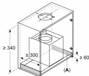
Matmenys, mm Montavimo reikalavimai, jei reikia ką nors pakeisti
