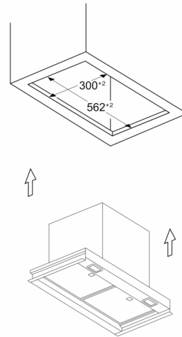
Matmenys, mm Montavimo pavyzdys su baldų išpjova
