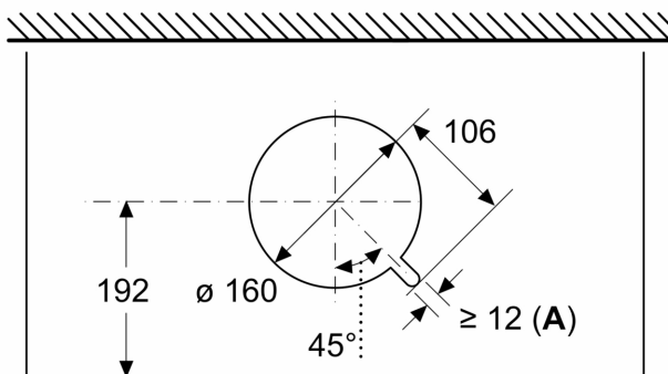
Matmenys, mm Vaizdas iš viršaus
