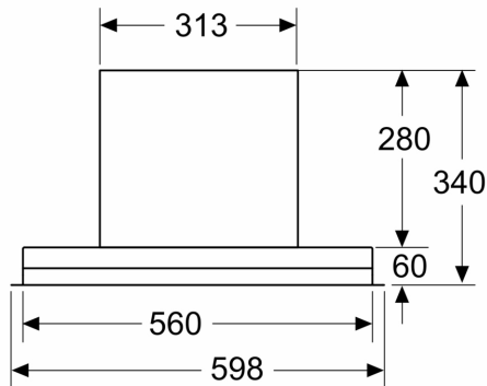
Matmenys, mm Vaizdas iš priekio
