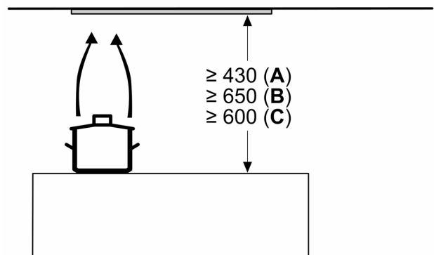
Matmenys, mm
