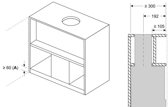
Matmenys, mm Montavimo pavyzdys su prieskonių lentyna
