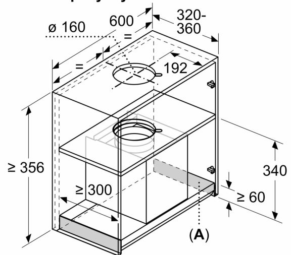
Matmenys, mm Montavimo pavyzdys
